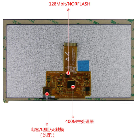
图 1-4 硬件配置图
