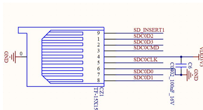
图 6-2SD 卡参考电路
