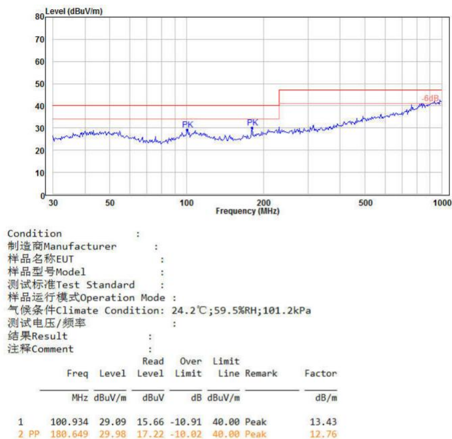
图 7-6 辐射测试水平方向
