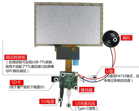
图 1-5 调试工具图
