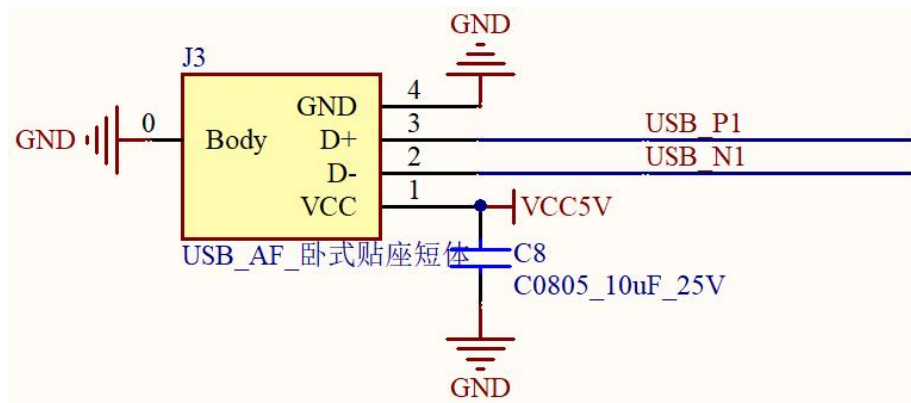
图 6-5U 盘参考电路
