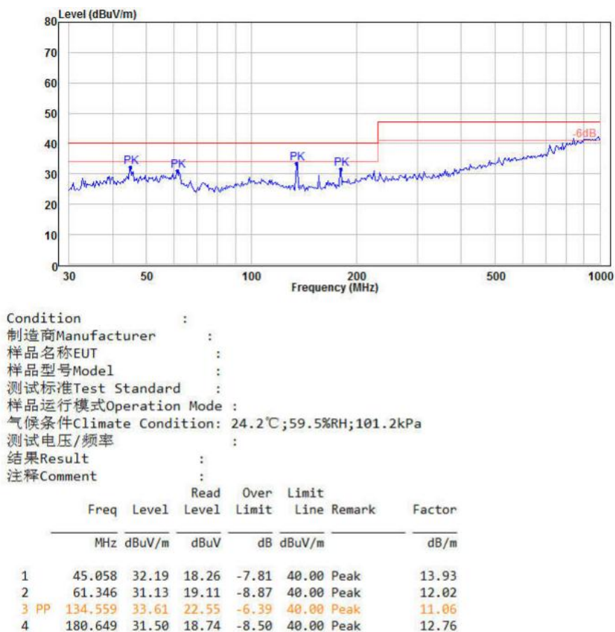
图 7-7 辐射测试垂直方向
